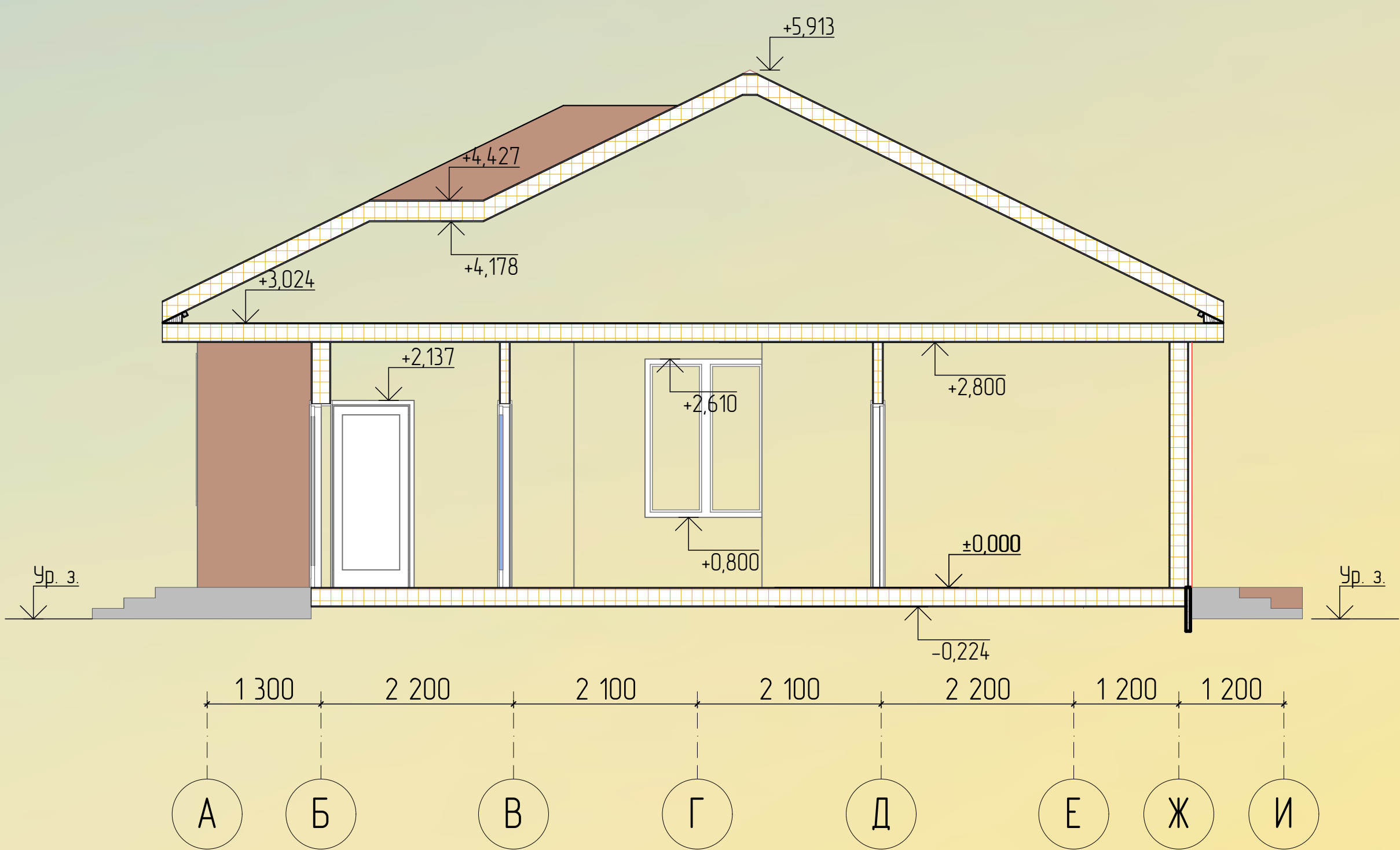
Разрез 1-1
